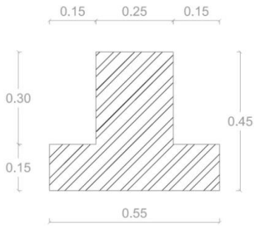
Εικόνα: Διατομή τοιχίου
