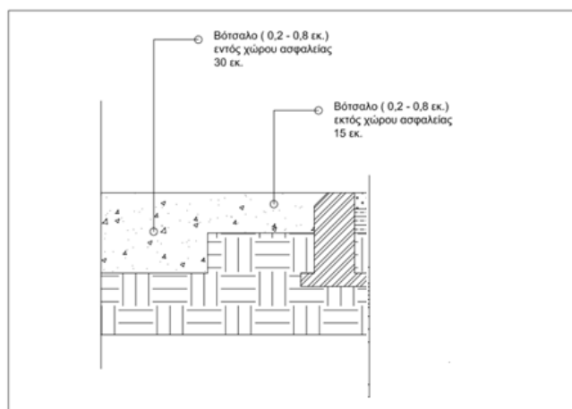
Εικόνα 1: Διατομή ενδεικτικής εφαρμογής φυσικού υλικού επίστρωσης δαπέδων ασφαλείας παιδικής χαράς Τιμή εφαρμογής: 69,00 €/ κ.μ.
