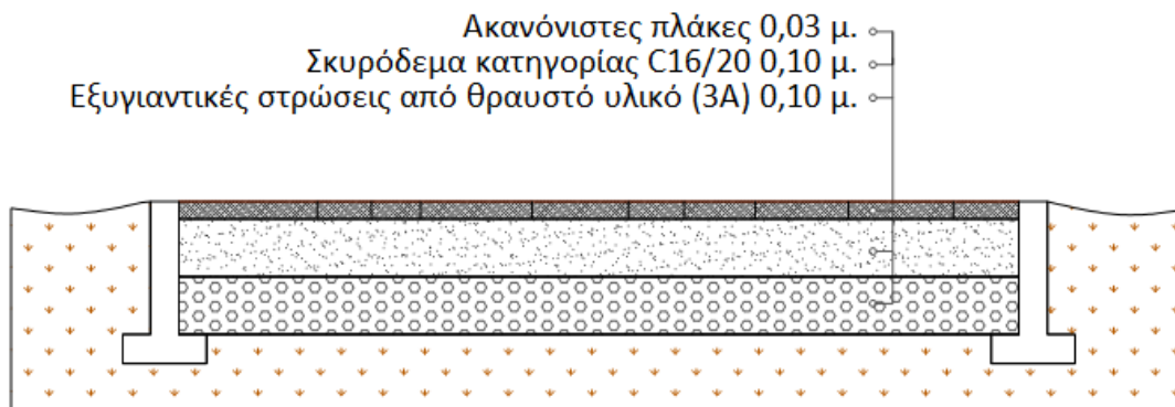
Εικόνα: Διατομή ενδεικτικής εφαρμογής δαπέδου που επιστρώνεται με ακανόνιστες πλάκες Τιμή εφαρμογής: 6,10 €/ τ.μ.
