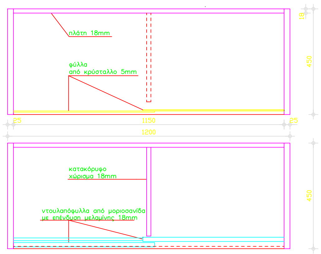
ΟΨΗ ΒΙΒΛΙΟΘΗΚΗΣ
