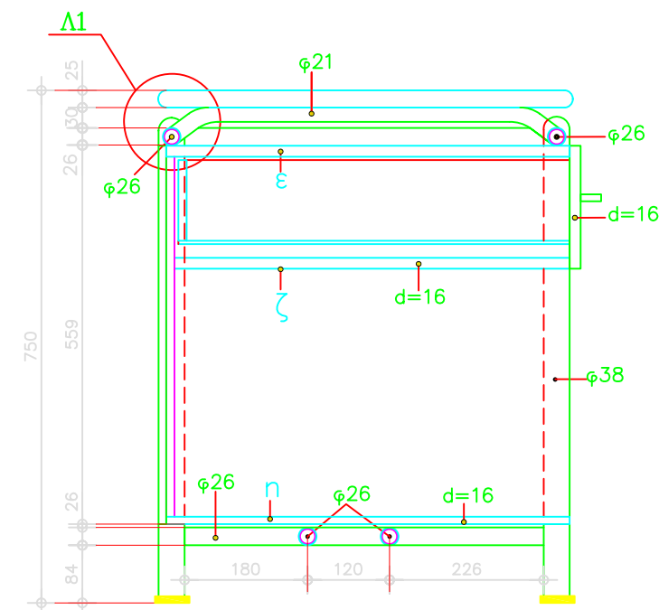
ΤΟΜΗ Δ-Δ
