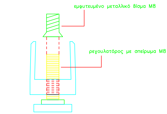
ΠΕΛΜΑ ΜΕ ΡΕΓΟΥΛΑΤΟΡΟ (Λ4)
