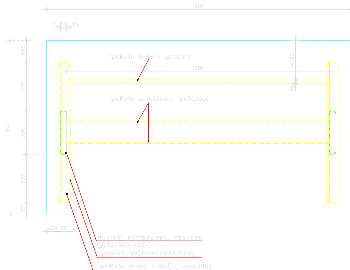
ΚΑΤΟΨΗ ΓΡΑΦΕΙΟΥ Η/Υ ΚΛ. 1:10
